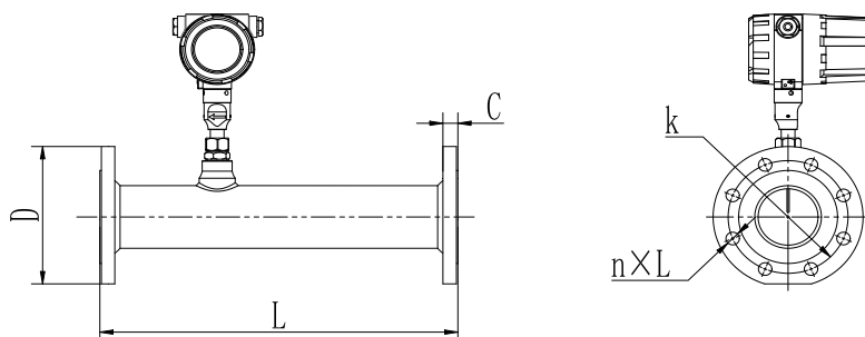
管段式安装尺寸
