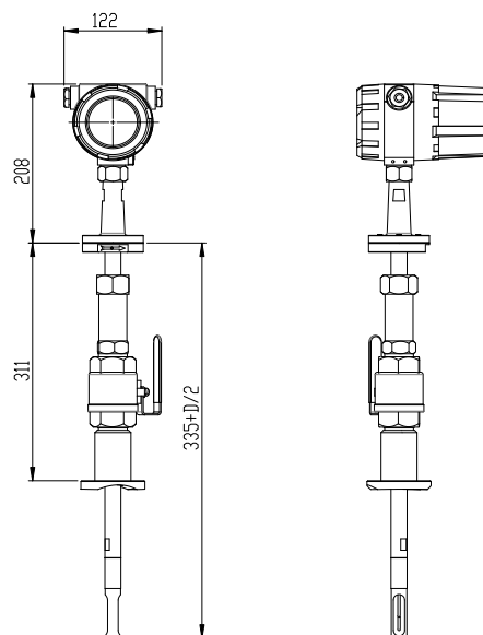
标准型外形尺寸
